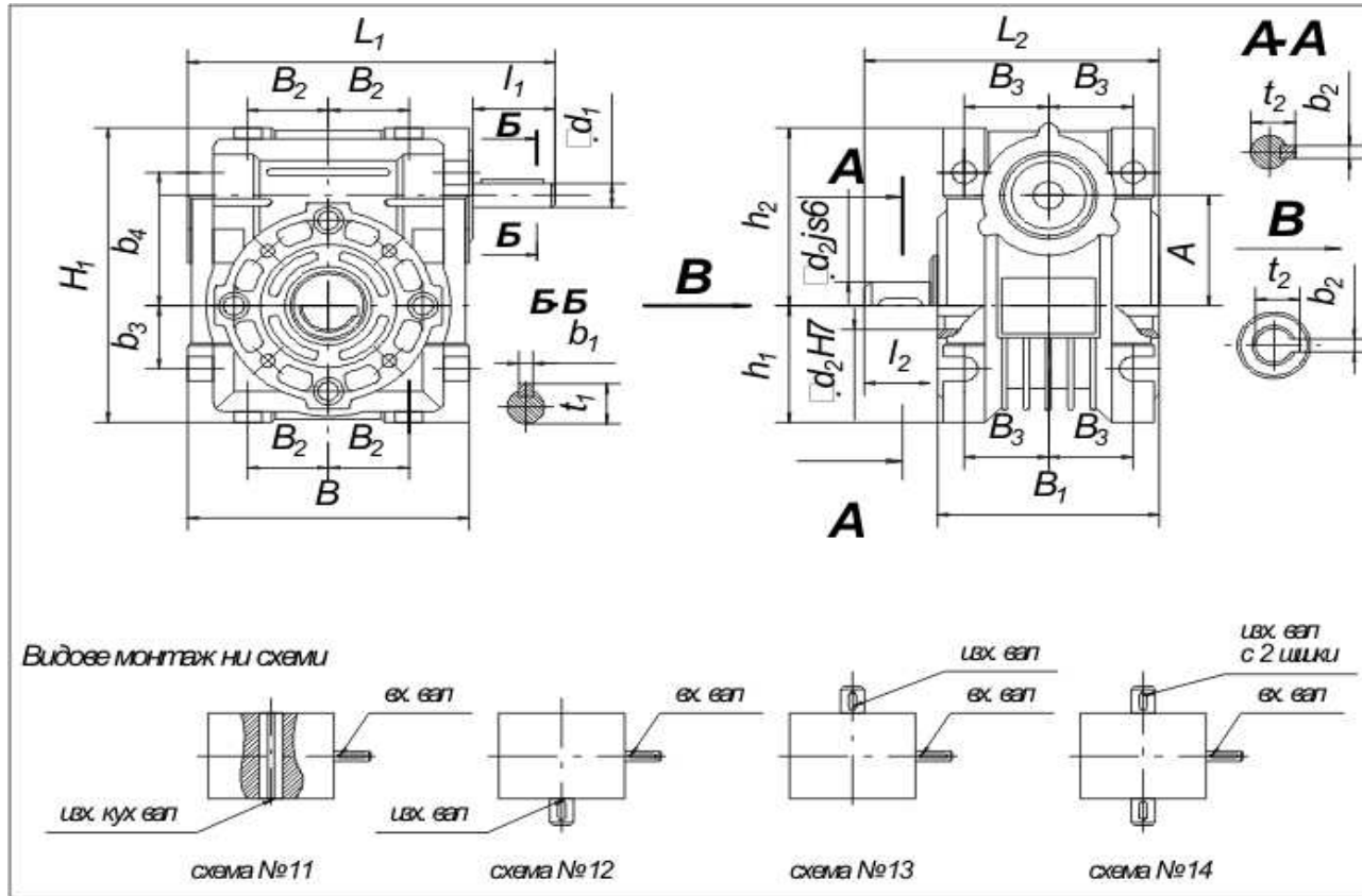
Присъединителни размери на редуктори червячни с олекотен алуминиев корпус
