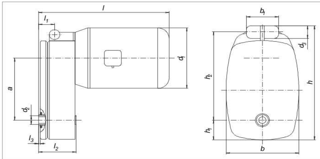
Редуктор - цилиндричен РЦ 305
