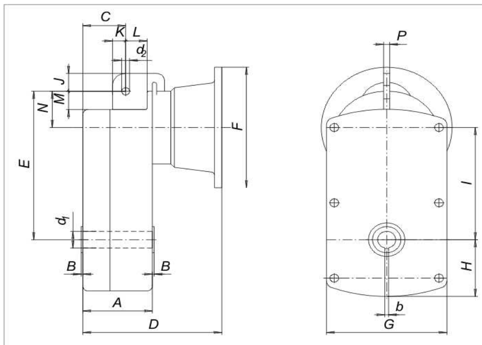
Трехступенчатые редукторы
